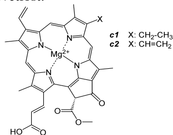
Slika 23.16. Struktura hlorofila
