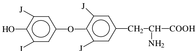
tiroksin
