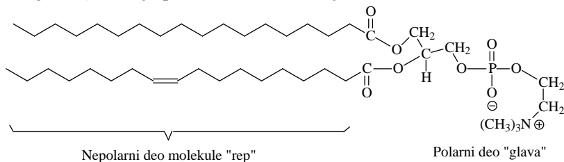
Slika 22.8. Bifilnost fosfoglicerida
