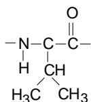
Valin (Val)
