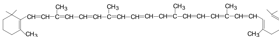
γ - karoten
