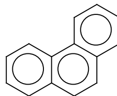
fenantren
