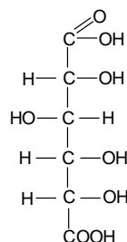
D-gluko-šećerna kiselina (aldarna)
