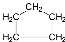
ciklopentan
