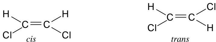
1,2-dihloretilen
