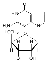
Guanozin G
