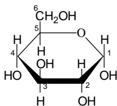
\alpha -D-glukopiranoza
