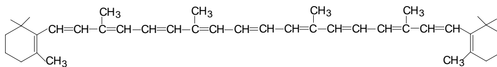
β - karoten
