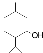
mentol (etarsko uljenane)
