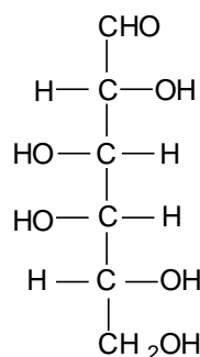
D-galaktoza
