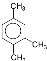
nesimetrični
