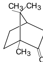
kamfor (kamforovo drvo)
