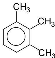
vicinalni
